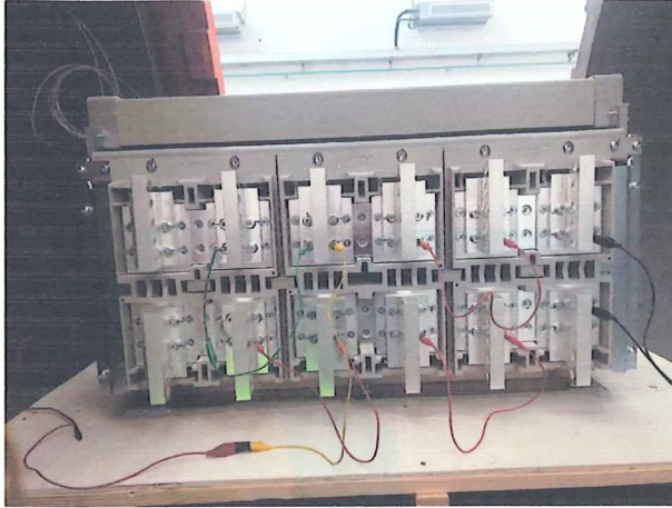
介电性能试验照片:
